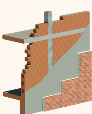
Figura 8. Fachada con hoja principal cerámica con un sistema prefabricado de aislamiento térmico por el exterior con acabado de plaqueta cerámica vista
