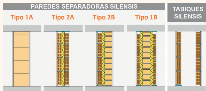
Figura 18. Tipos de paredes separadoras y tabiques Silensis
