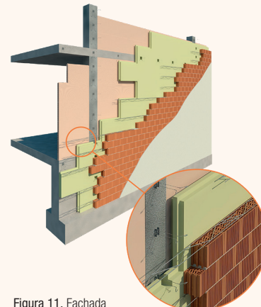
Figura 11. Fachada autoportante de dos hojas de fábrica
